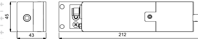
CM Tiny 技术图纸
